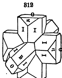
Staurolite.
